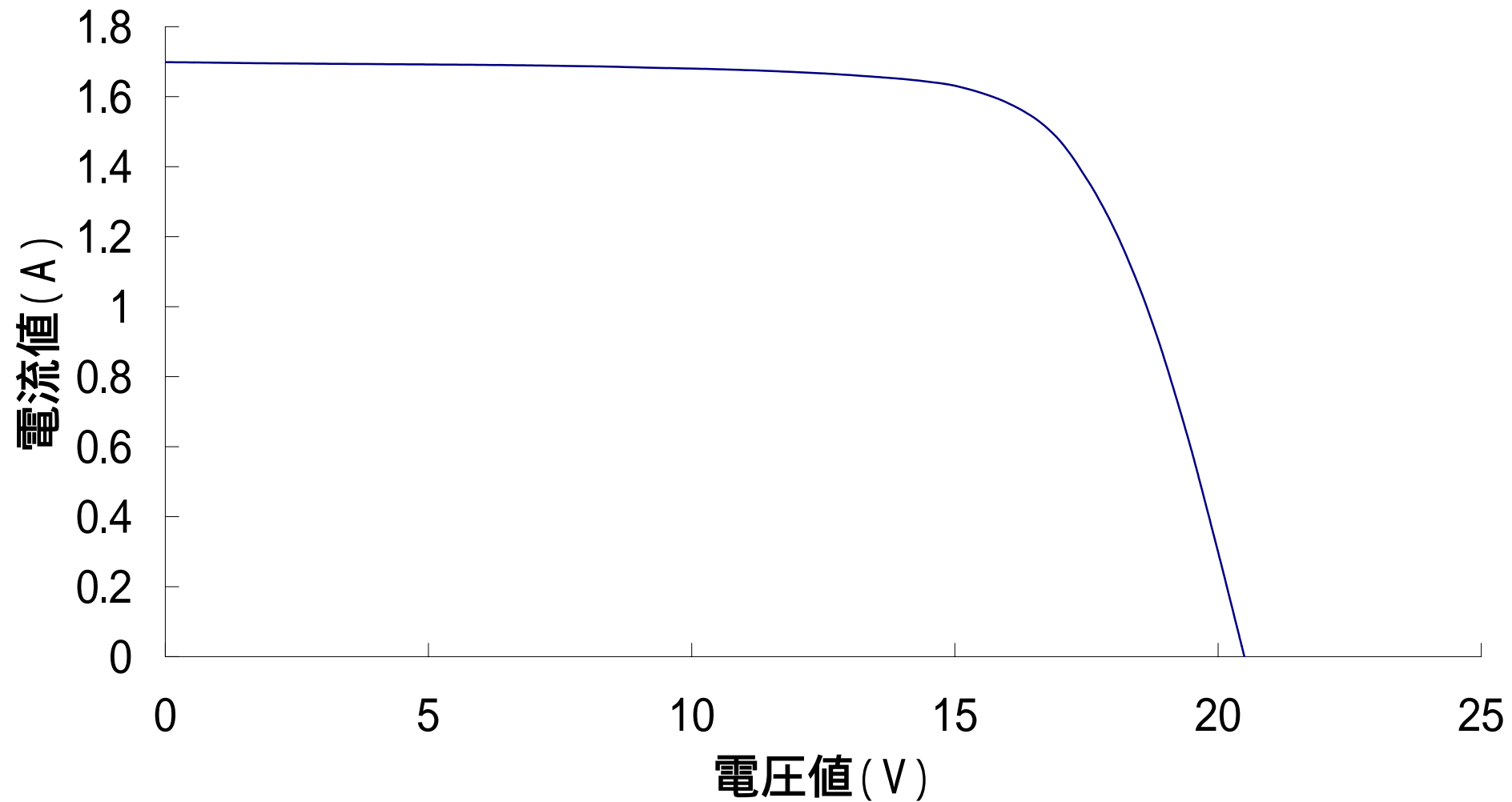
GT 2 3 4 出力特性図 @1000W/m 2 AM1.5 25
